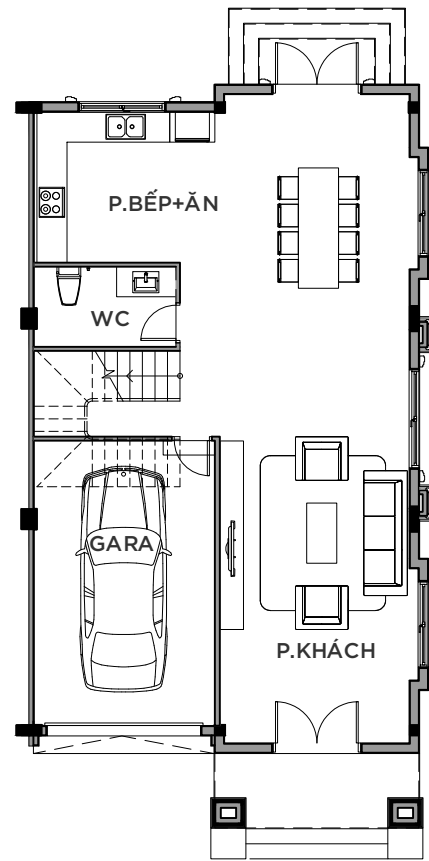
MẶT BẰNG TẦNG 1
