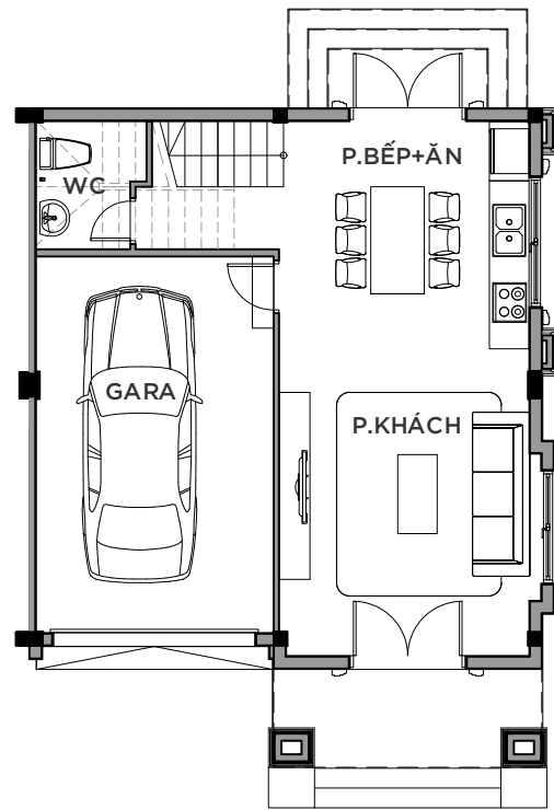
MẶT BẰNG TẦNG 1
