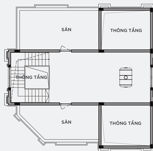
MẶT BẰNG ÁP MÁI
