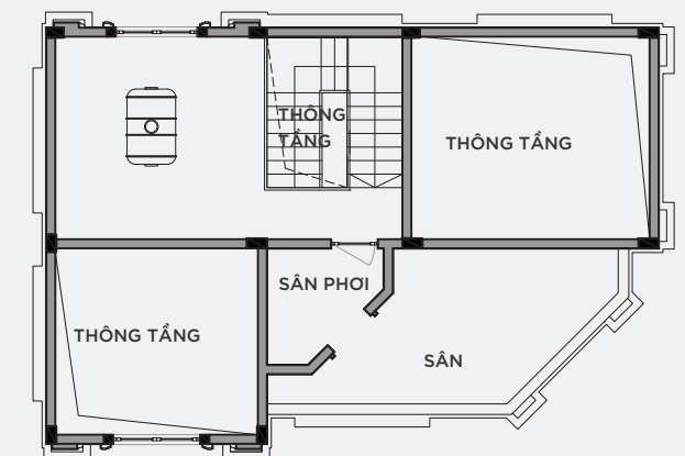
MẶT BẰNG ÁP MÁI
