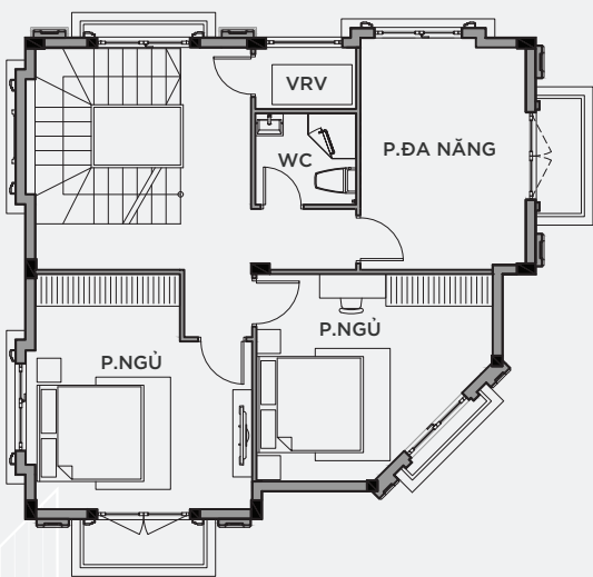
MẶT BẰNG TẦNG 3
