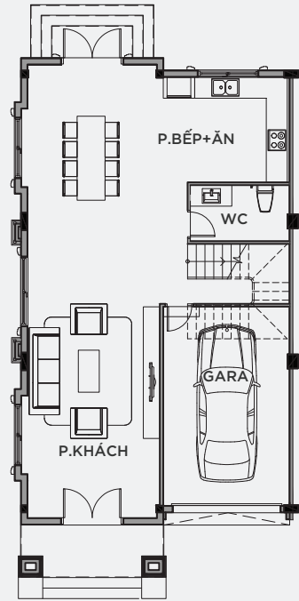
MẶT BẰNG TẦNG 1
