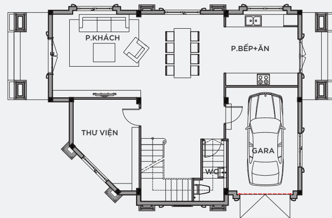
MẶT BẰNG TẦNG 1
