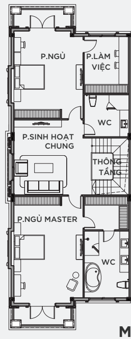
MẶT BẰNG TẦNG 1
