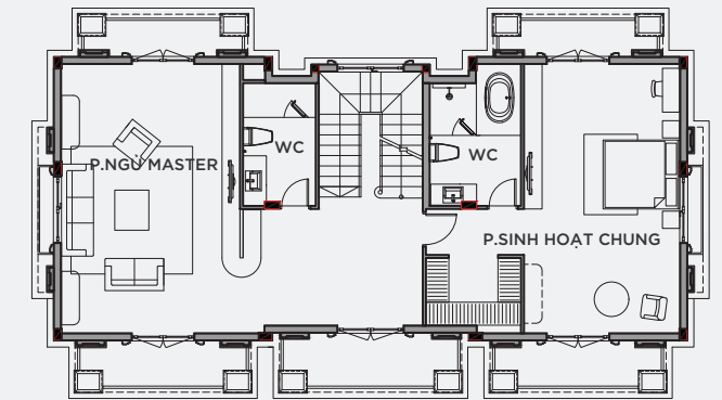
MẶT BẰNG TẦNG 2
