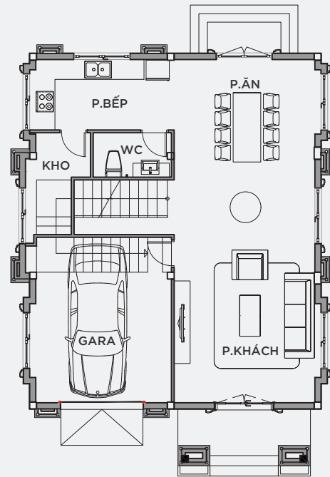
MẶT BẰNG TẦNG 1
