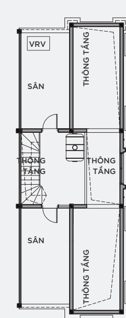
MẶT BẰNG ÁP MÁI
