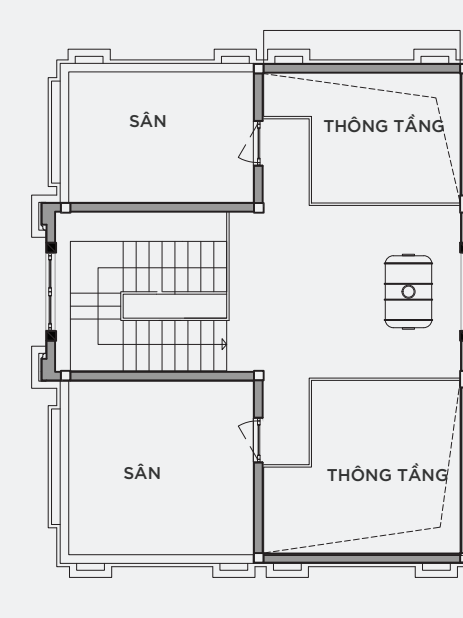
MẶT BẰNG ÁP MÁI
