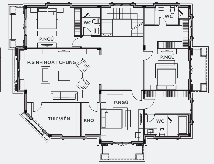
MẶT BẰNG TẦNG 2
