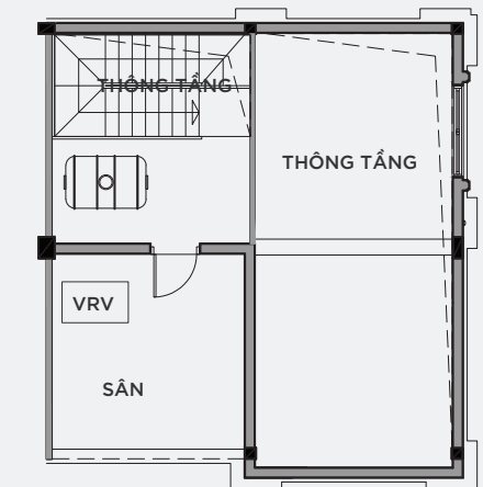
MẶT BẰNG ÁP MÁI
