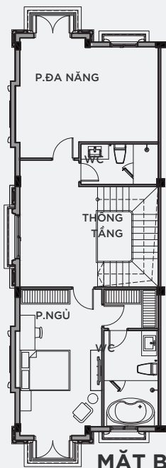
MẶT BẰNG TẦNG 1
