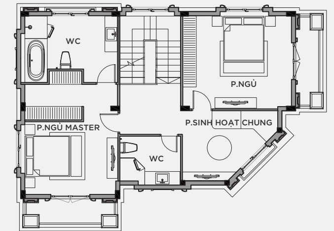
MẶT BẰNG TẦNG 2
