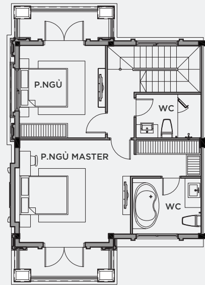
MẶT BẰNG TẦNG 2
