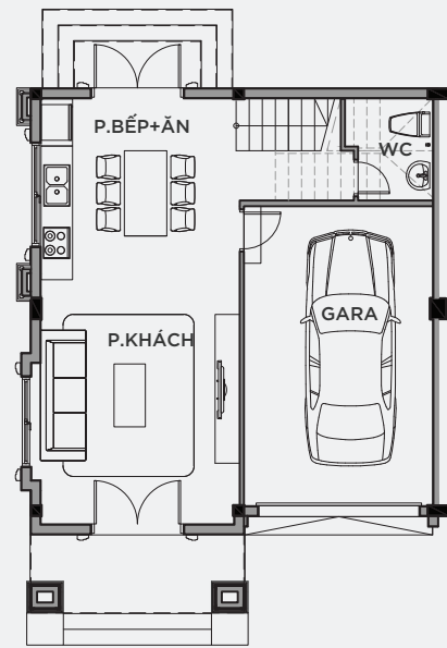
MẶT BẰNG TẦNG 1
