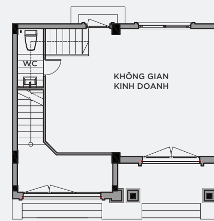
MẶT BẰNG TẦNG 1
