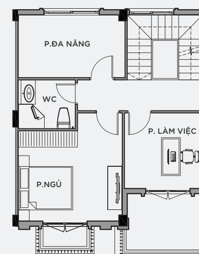
MẶT BẰNG TẦNG 5
