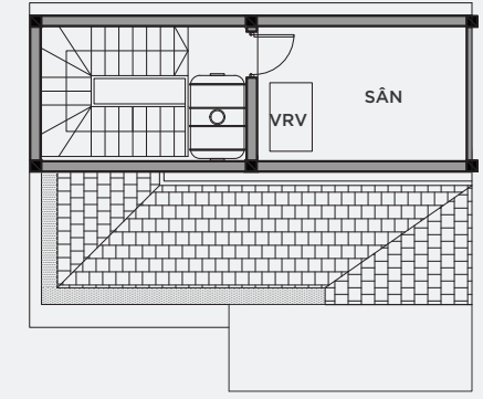
MẶT BẰNG ÁP MÁI
