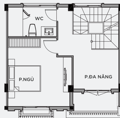
MẶT BẰNG TẦNG 5
