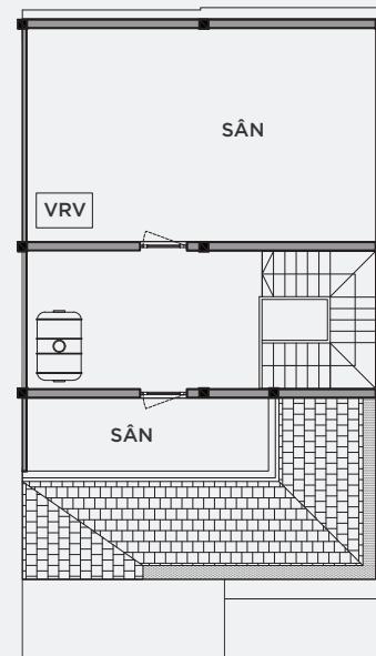
MẶT BẰNG ÁP MÁI
