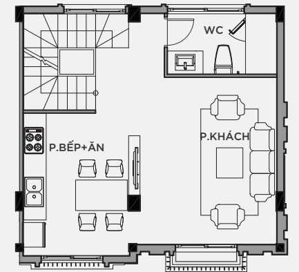
MẶT BẰNG TẦNG 3
