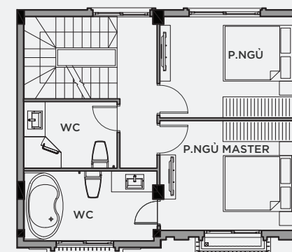
MẶT BẰNG TẦNG 4
