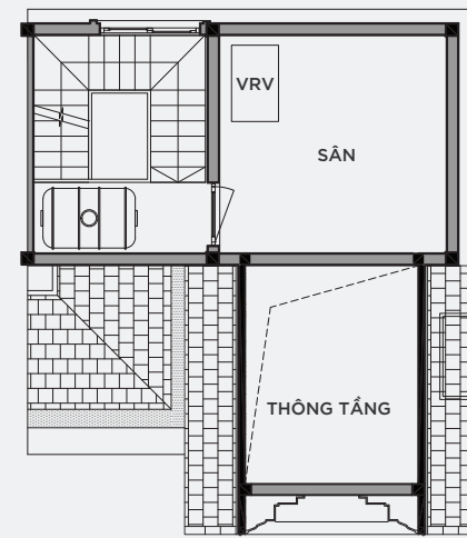
MẶT BẰNG ÁP MÁI
