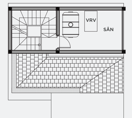
MẶT BẰNG ÁP MÁI
