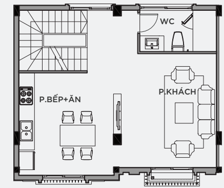
MẶT BẰNG TẦNG 3
