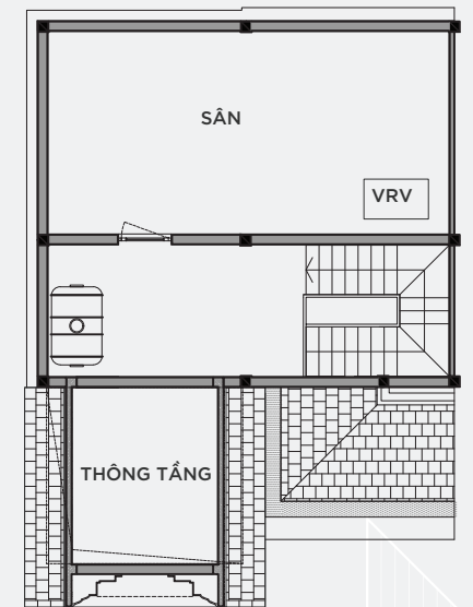
MẶT BẰNG ÁP MÁI
