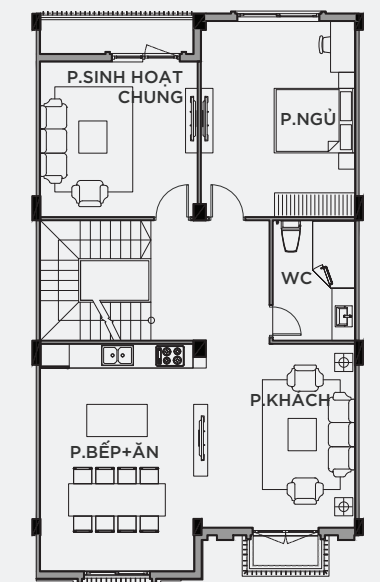
MẶT BẰNG TẦNG 3
