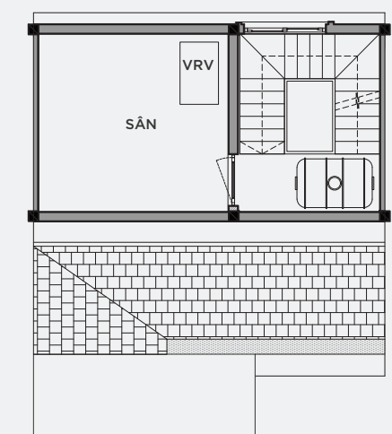
MẶT BẰNG ÁP MÁI
