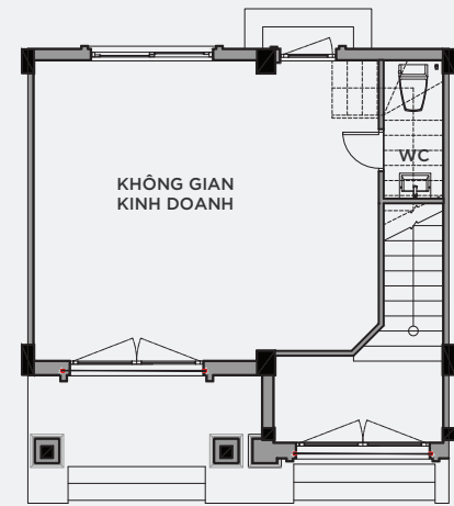
MẶT BẰNG TẦNG 1
