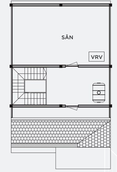
MẶT BẰNG ÁP MÁI
