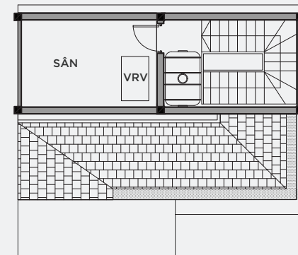
MẶT BẰNG ÁP MÁI
