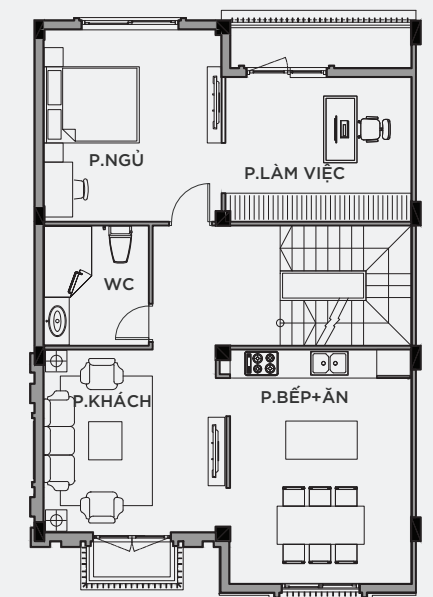
MẶT BẰNG TẦNG 3
