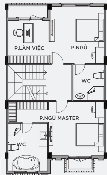
MẶT BẰNG TẦNG 4
