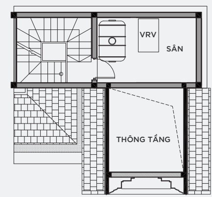
MẶT BẰNG ÁP MÁI
