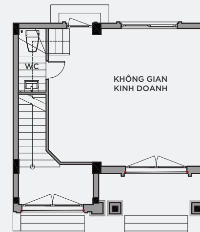
MẶT BẰNG TẦNG 1
