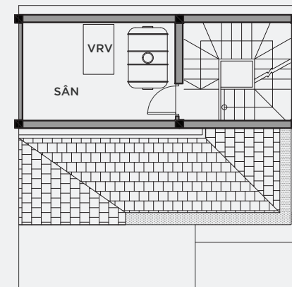
MẶT BẰNG ÁP MÁI
