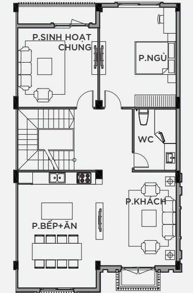
MẶT BẰNG TẦNG 3
