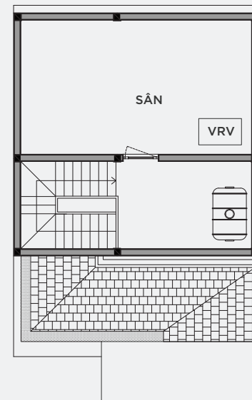
MẶT BẰNG ÁP MÁI
