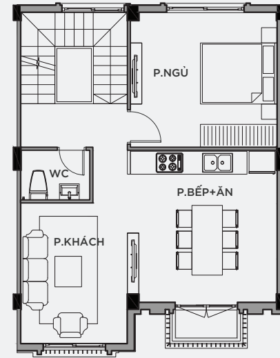
MẶT BẰNG TẦNG 3
