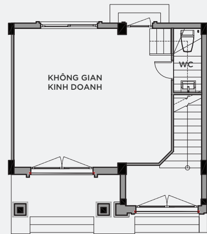
MẶT BẰNG TẦNG 1
