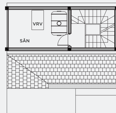
MẶT BẰNG ÁP MÁI
