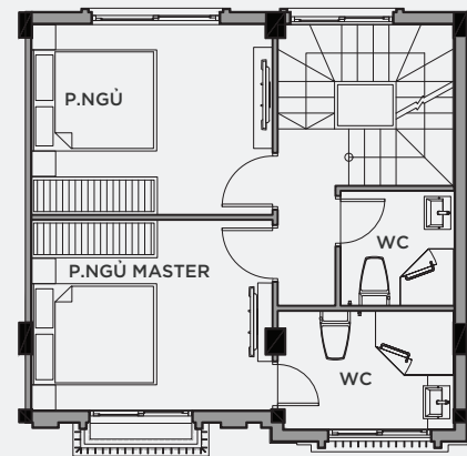
MẶT BẰNG TẦNG 4
